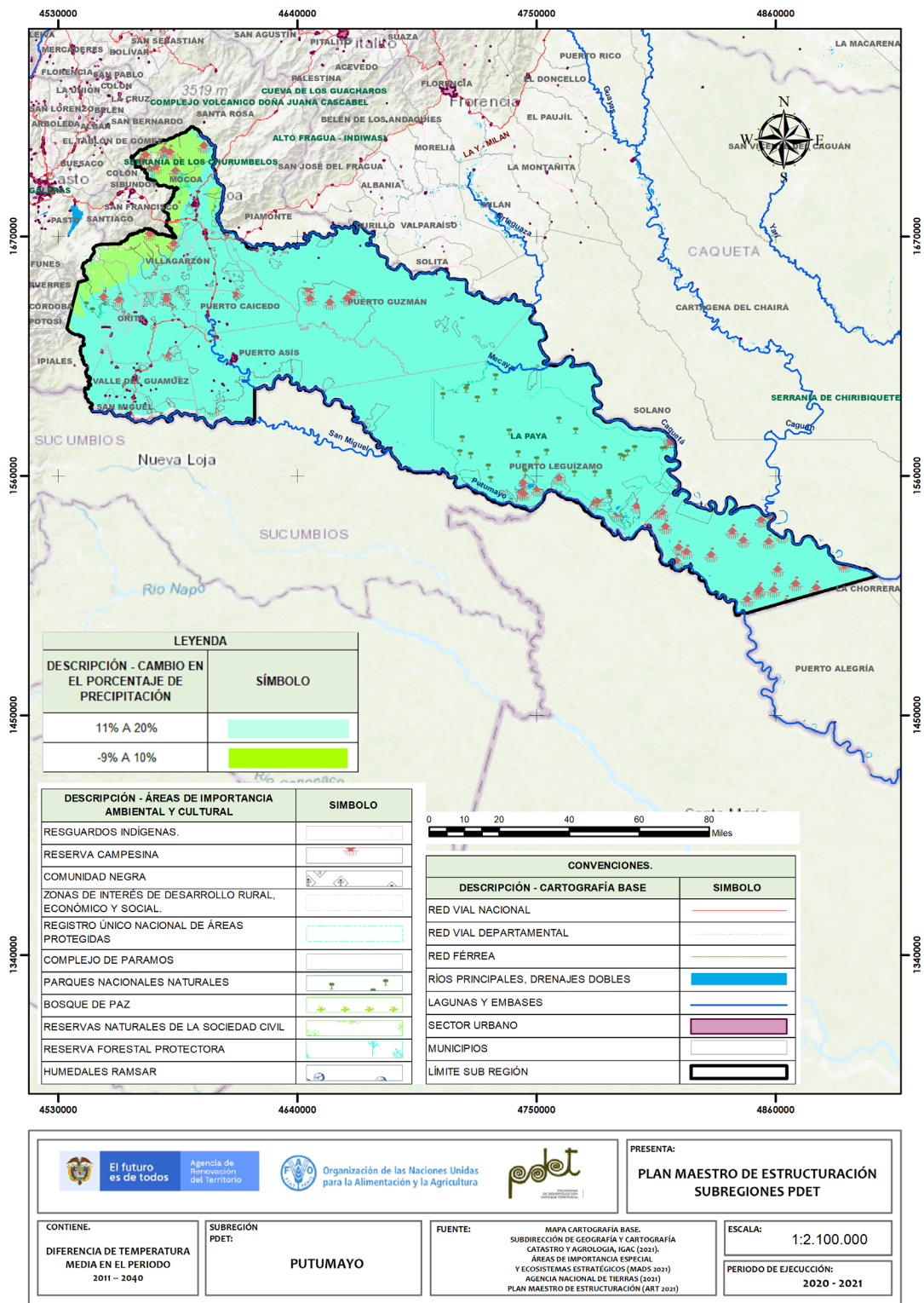
Ilustración 3. Escenario RPC 6.0 de cambio climático para 2040 para la precipitación promedio y la temperatura media para la subregión PDET Putumayo
