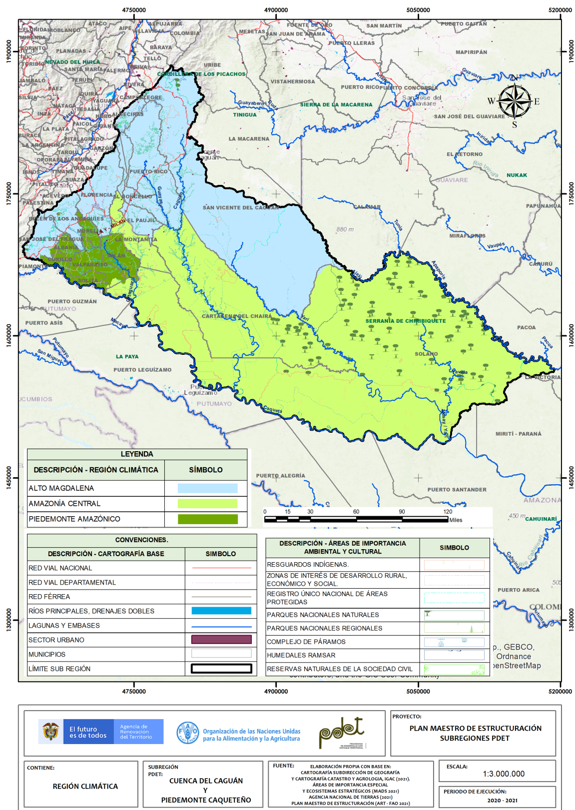
Ilustración 1. Regiones climáticas para la subregión
