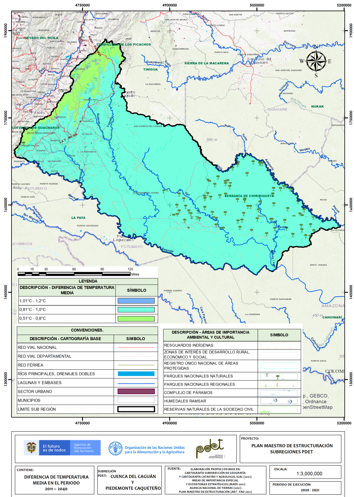
Ilustración 3. Escenario RPC 6.0 de cambio climático para 2040 para la precipitación promedio y la temperatura media para la subregión PDET Cuenca del Caguán y Piedemonte Caqueteño
