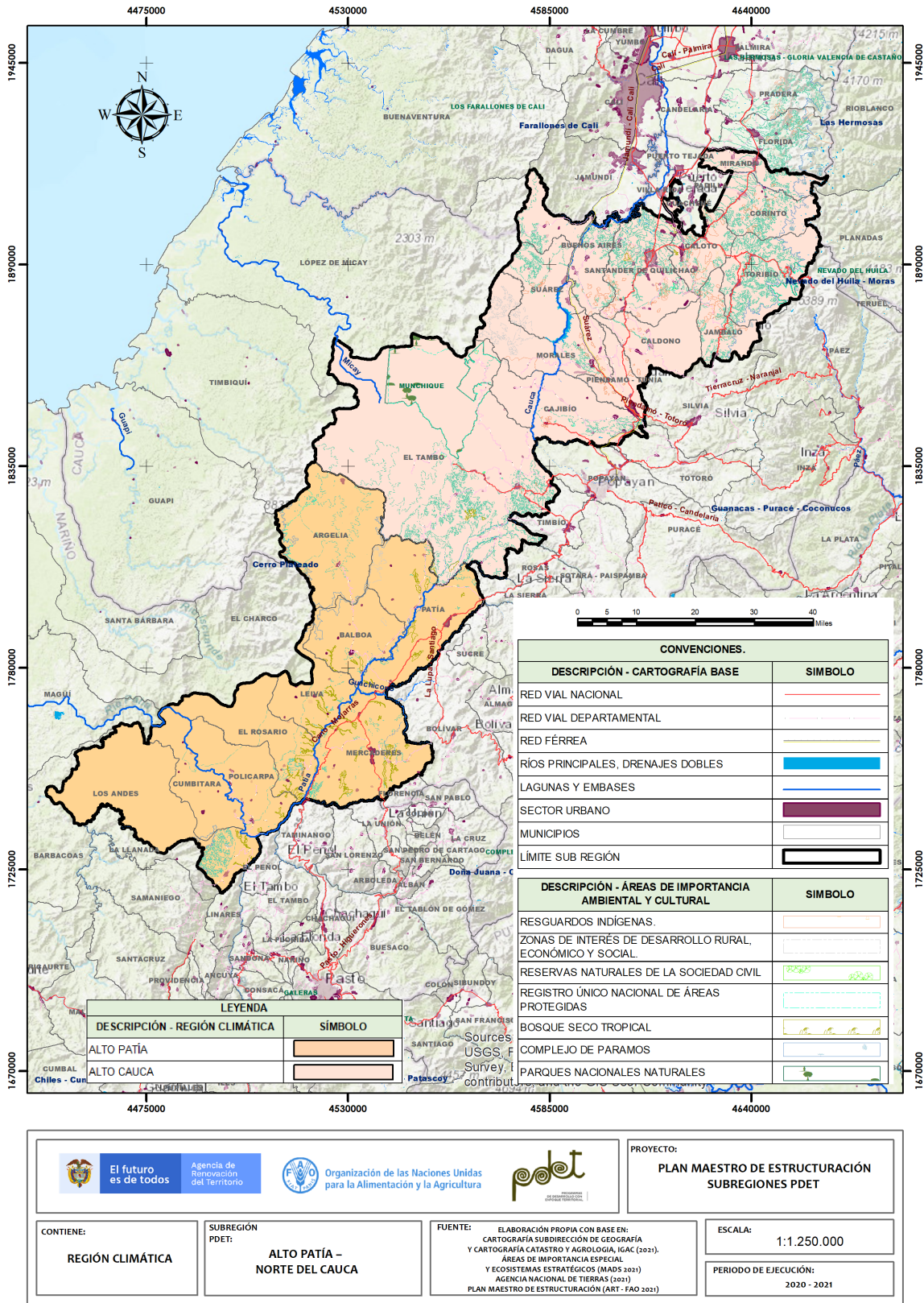
Ilustración 1. Regiones climáticas para la subregión PDET Alto Patía - Norte del Cauca
