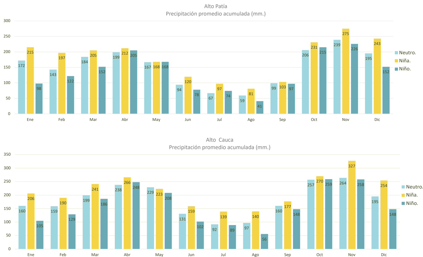
Ilustración 2. Influencia en la precipitación de los fenómenos de variabilidad climática de El Niño–La Niña respecto al promedio de los años neutros para el periodo 1975–2015. En la parte inferior del gráfico los meses están representados por sus iniciales.
